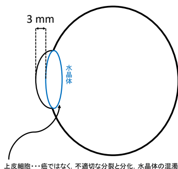
図 4.12: 目の模式図
