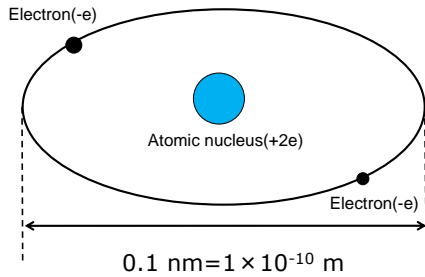
図 1.4: 原子模型
