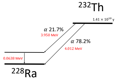
図 3.6: トリウム 232
