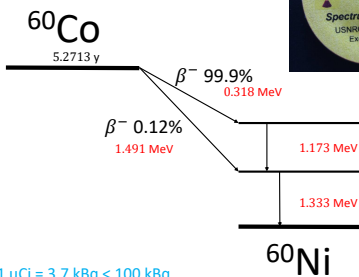
図 3.7: コバルト 60
