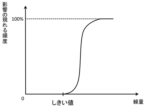
図 4.2: 確定的影響
