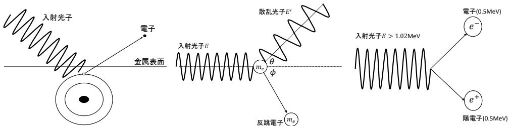
図 2.15: 光電効果
