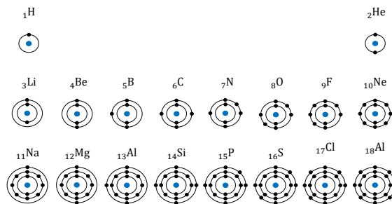
図 1.7: 周期表
