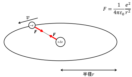
図 1.5: ボーア模型
