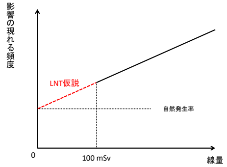
図 4.3: 確率的影響
