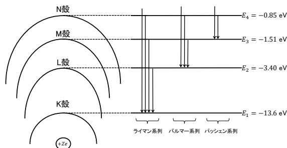
図 1.9: 特性 X 線
